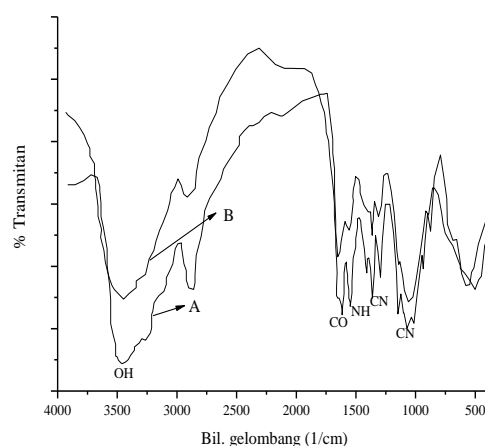
Gambar.1. Spektra IR kitosan serbuk (A) dan kitosan bead (B)
