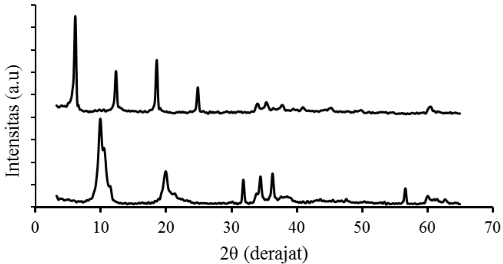
Gambar 1. XRD polikristalin hidrotalsit Zn-Al; (a) hidrotalsit Zn-Al- \text{NO}_3 dan (b) hidrotalsit Zn-Al-EDTA
