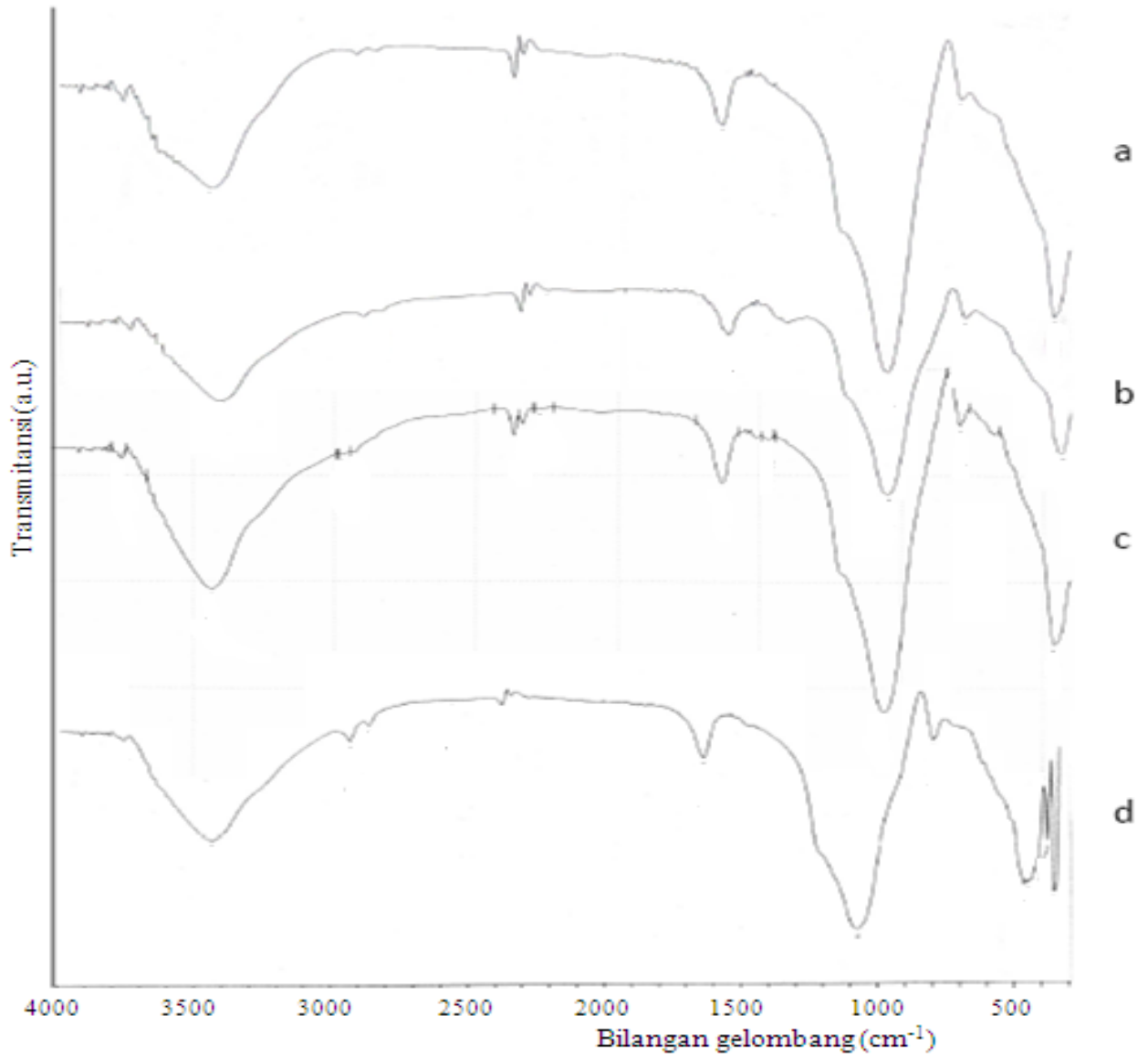
Gambar 1. Spektra inframerah sampel zeolit, yaitu (a) zeolit alam, (b) zeolit teraktivasi asam, (c) zeolit termodifikasi CTAB dan (d) zeolit termodifikasi propilamin.
