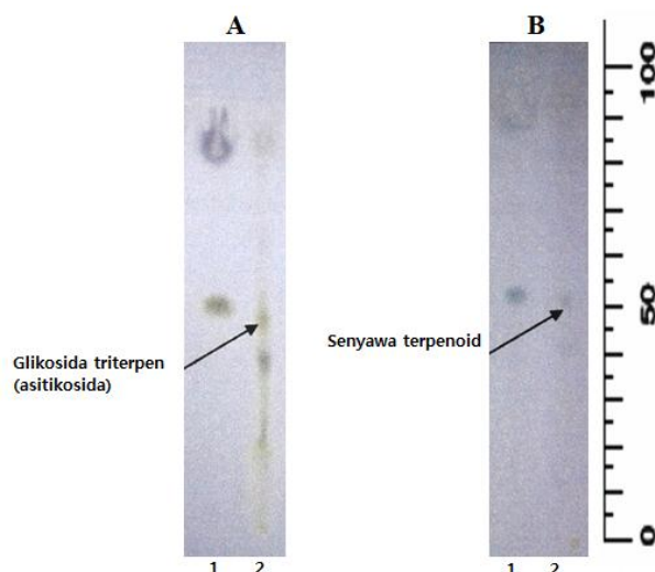
Gambar 3. Hasil identifikasi senyawa asiaticosida menggunakan KLT dengan pereaksi vanilin asam sulfat (A) dan pereaksi LB (B). Terlihat bercak ekstrak pegagan (1) dan bercak dari pembanding TECA ( tritared extract Centella asiatica ) sebagai standar (2).
