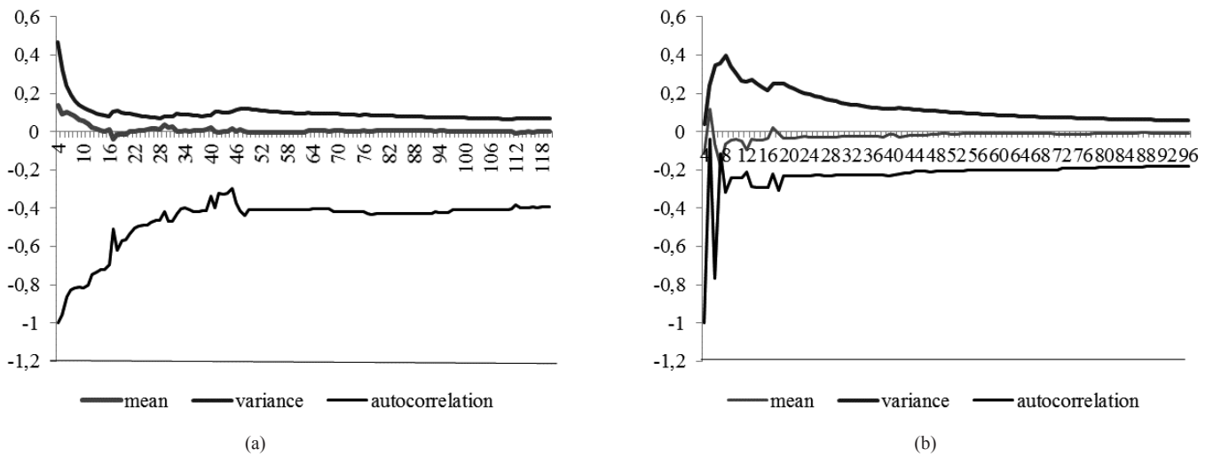
Gambar 6. Mean, variance, dan autokorelasi data debit Sungai Bedog (a) dan Gajahwong (b) setelah proses differencing lag 1
