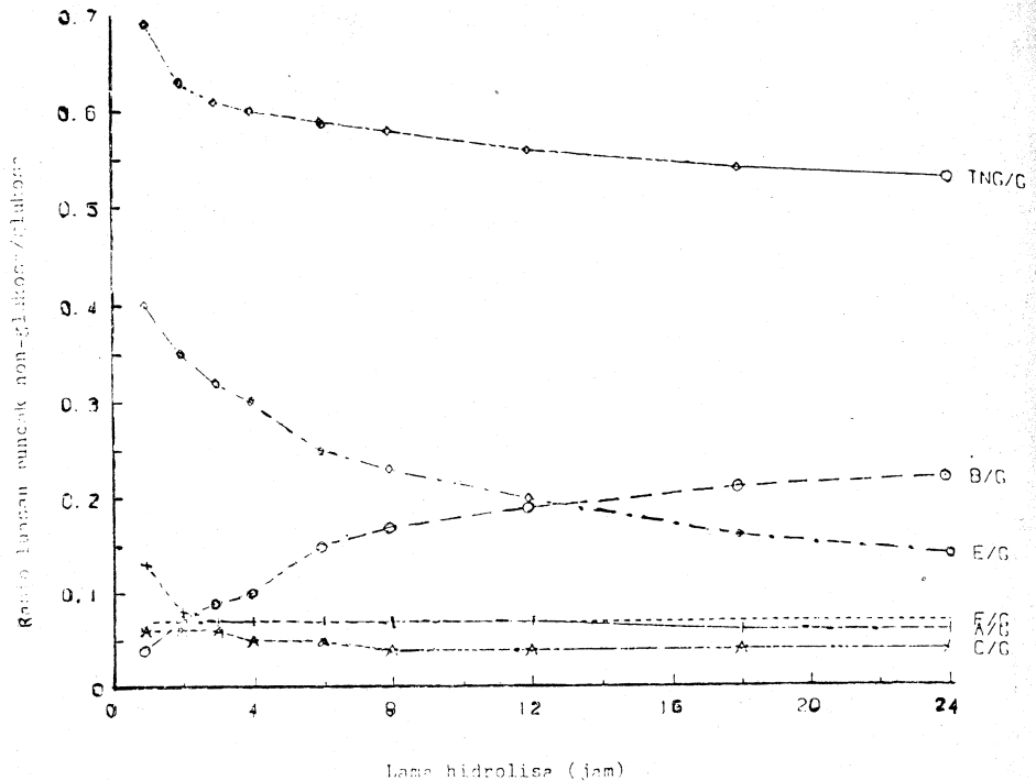
Gambar 2. Pengaruh lama hidrolisa terhadap rasio luasan puncak-puncak non-glukosa terhadap dan puncak glukosa dari kromatogram-kromatogram hidrolisat pati hidroksipropil
