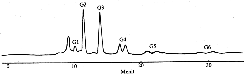
Gambar 1. Oligosakarida dari hidrolisis pati hidroksipropil dengan PPA, dipisahkan dengan HPLC menggunakan kolom \mu Bondapak.
