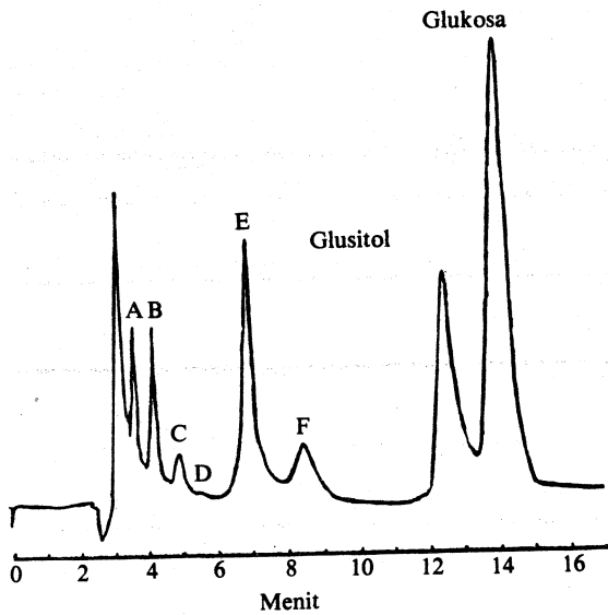
Gambar 2. Hasil hidrolisis asam dari hidrolisat PPA tereduksi dipisahkan dengan kolom \mu Poracil.
