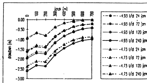
Gambar 10. Penurunan aras airtanah dengan pola operasi 9 pompa berjarak 200 m
