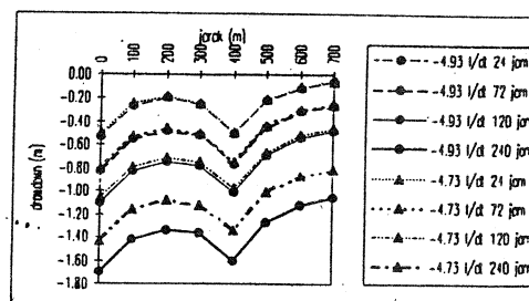
Gambar 11. Penurunan aras airtanah dengan pola operasi 9 pompa berjarak 400 m
