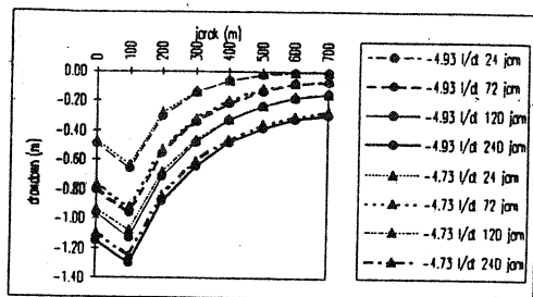
Gambar 8. Penurunan aras airtanah dengan pola operasi 4 pompa berjarak 200 m
