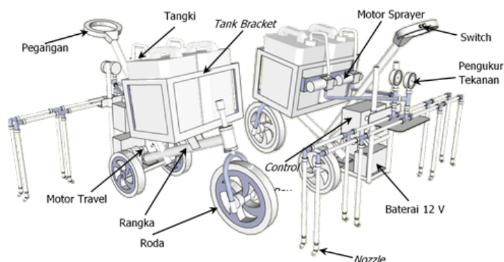
Gambar 1. Aplikator pupuk terkontrol atau Variable-Rate Application (VRA)
