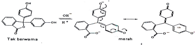
Gambar 2. Bentuk kestimbangan dari fenolftalein
