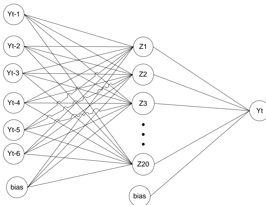
Gambar 2 Arsitektur jaringan
