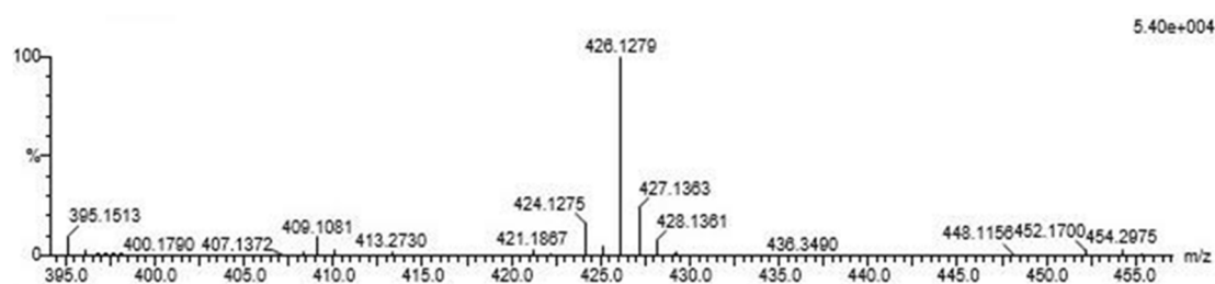
Fig S17. HRMS spectrum of 4e
