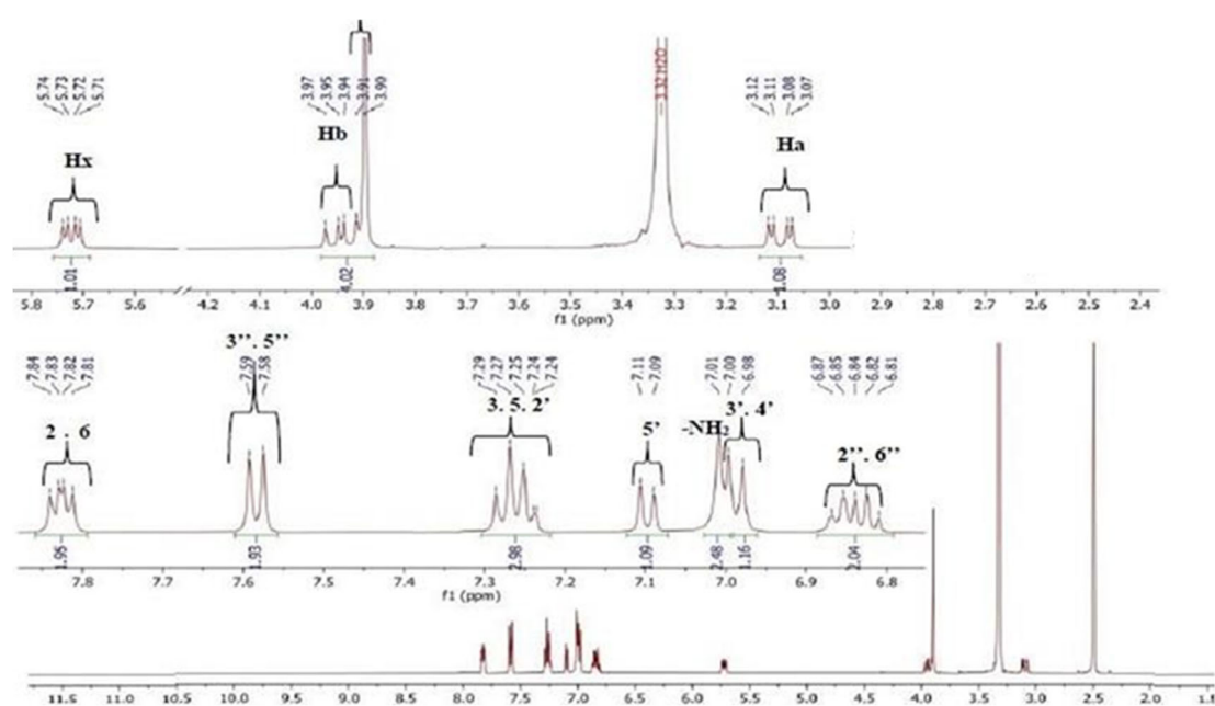
Fig S18. 1 H-NMR spectrum of 4e
