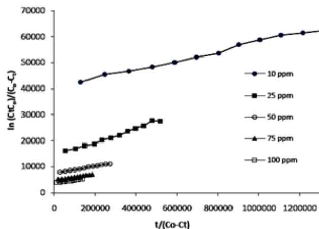
Gambar 5. Kurva hubungan \{\ln (C_o/C_t)\}/(C_o-C_t) versus t/(C_o-C_t) untuk adsorpsi Cd(II) oleh adsorben untuk konsentrasi awal Cd(II) 10 hingga 100 ppm
