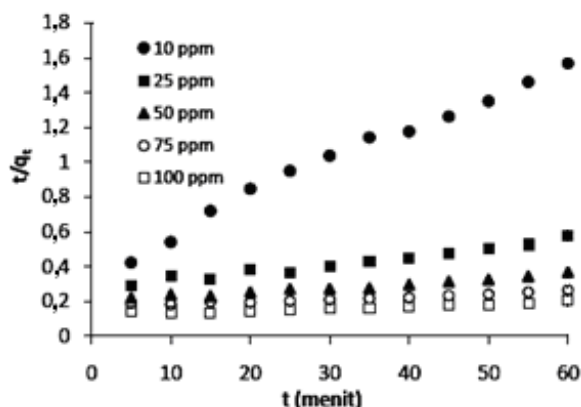
Gambar 11. Kurva hubungan t/q_t versus t untuk adsorpsi Cd(II) oleh adsorben pada konsentrasi awal Cd(II) 10 hingga 100 ppm
