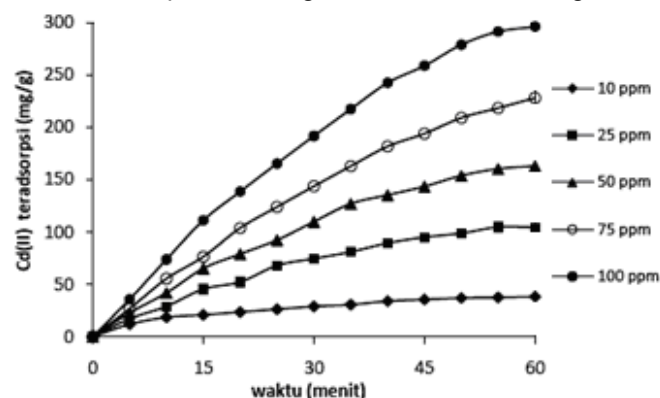
Gambar 2. Kurva hubungan Cd(II) teradsorpsi dengan waktu reaksi pada berbagai konsentrasi awal logam
