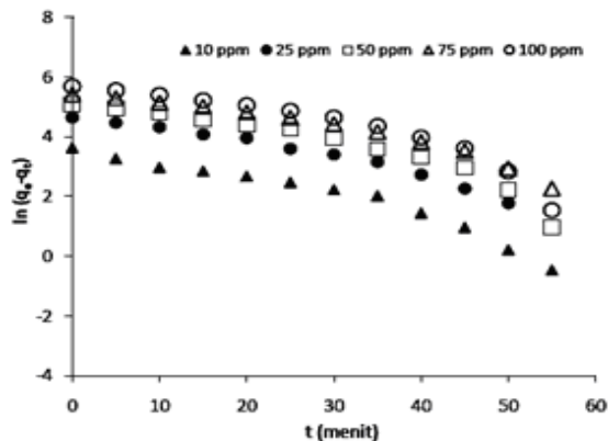
Gambar 8. Kurva hubungan \ln (q_e-q_t) versus t untuk adsorpsi Cd(II) pada adsorben untuk konsentrasi awal Cd(II) 10 hingga 100 ppm
