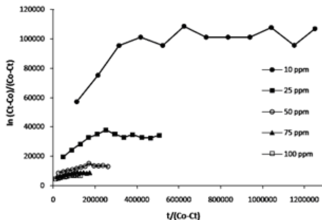
Gambar 4. Kurva hubungan \{\ln (C_o/C_t)\}/(C_o-C_t) versus t/(C_o-C_t) untuk adsorpsi Pb(II) oleh adsorben pada konsentrasi awal Pb(II) 10 hingga 100 ppm
