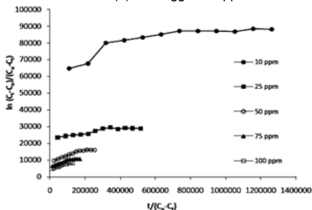
Gambar 6. Kurva hubungan \{\ln (C_o/C_t)\}/(C_o-C_t) versus t/(C_o-C_t) untuk adsorpsi Cr(III) oleh adsorben untuk konsentrasi awal Cr(III) 10 hingga 100 ppm
