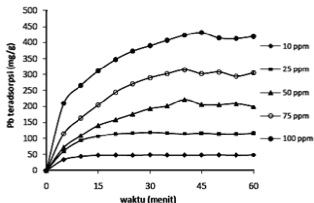
Gambar 1. Kurva hubungan Pb(II) teradsorpsi dengan waktu reaksi pada berbagai konsentrasi awal logam
