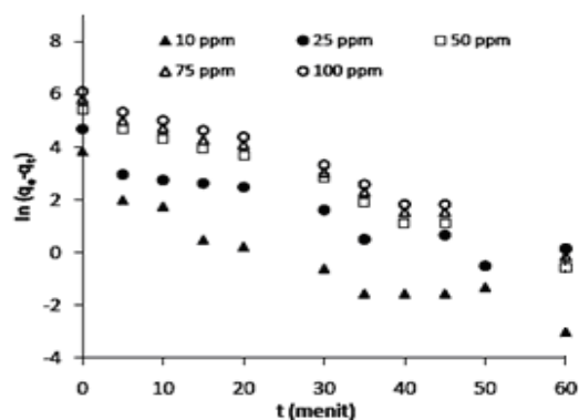
Gambar 9. Kurva hubungan \ln (q_e - q_t) versus t untuk adsorpsi Cr(III) pada adsorben untuk konsentrasi awal Cr(III) 10 hingga 100 ppm
