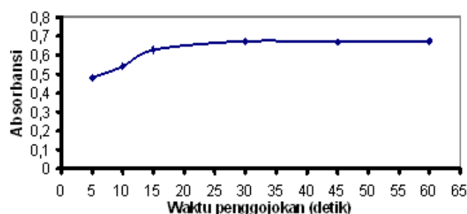
Gambar 5. Waktu ekstraksi kompleks 4-(4-nitrobenzenazo)-1-aminonaftalen ke dalam pelarut n-amilalkohol pada kadar nitrit 0,02 mg/L \text{N-NO}_2^- dengan pemekatan 10 kali.
