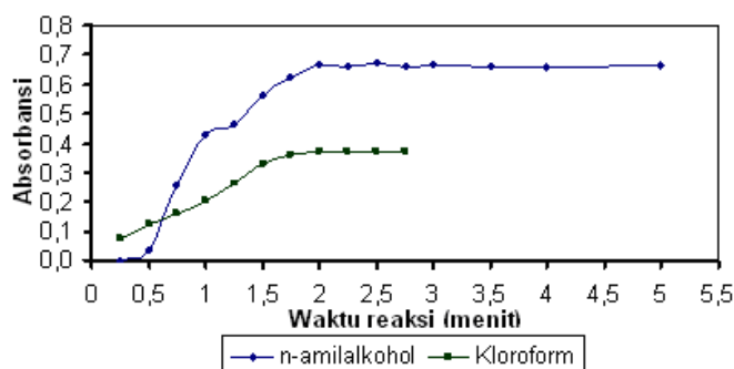
Gambar 4. Kurva waktu reaksi lawan absorbansi pada pembentukan kompleks 4-(4-nitrobenzenazo)-1-aminonaftalen dengan konsentrasi nitrit dalam air 0,02 mg/L (sebagai N) dan pemekatan 10 kali dalam n-amilalkohol dan kloroform.
