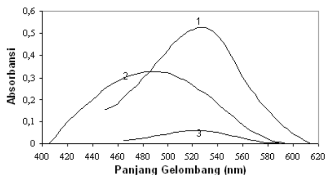
Gambar 2. Spektra absorpsi pada daerah tampak untuk kompleks produk reaksi diazotisasi-kopling dengan 4-nitroanilin dan 1-aminonaftalen pada konsentrasi nitrit 0,02 mg/L N-NO_2^- dalam n-amilalkohol (1), kloroform (2), dan air (3).
