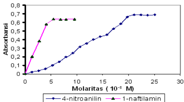
Gambar 7. Pengaruh konsentrasi pereaksi terhadap pembentukan kompleks 4-(4-nitrobenzenazo)-1-amino naftalen setelah pemekatan 10 kali dalam pelarut n-amilalkohol pada 0,02 mg/L N-NO 2 - .
