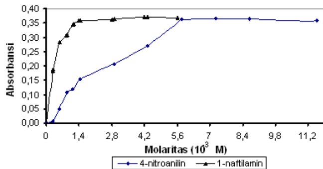
Gambar 8. Pengaruh konsentrasi 4-nitroanilin dan 1-aminonaftalen terhadap pembentukan kompleks 4-(4-nitrobenzenazo)-1-aminonaftalen dalam pelarut kloroform pada 0,02 mg/L N-NO 2 - dengan pemekatan 10 kali.
