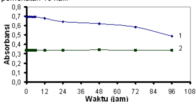
Gambar 6. Waktu kestabilan kompleks 4-(4-nitrobenzenazo)-1-aminonaftalen (1) dalam n-amilalkohol, dan (2) dalam kloroform setelah pemekatan 10 kali dari 0,02 mg/L \text{N-NO}_2^- dalam air.
