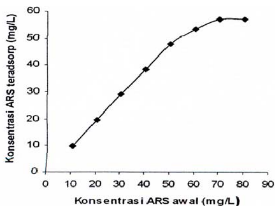
Gambar 9. Pengaruh konsentrasi awal ARS terhadap kemampuan adsorpsi.
