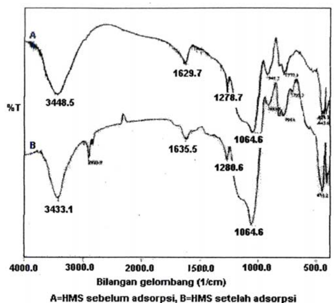
Gambar 10. Spektra perbandingan HMS sebelum dan setelah adsorpsi.
