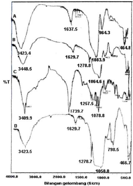
Gambar 3. Spektra inframerah SG dan HMS. A = SG, B = HMS, C = HMS dengan TA, D = HMS dengan TA setelah ekstraksi
