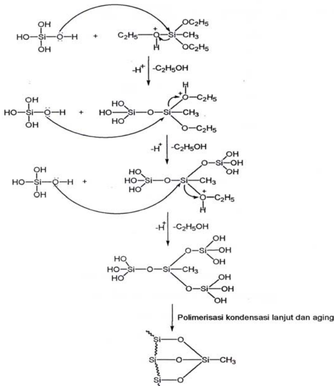
Gambar 1. Mekanisme reaksi pembentukan HMS dari prekursor TEOS dan MTES.
