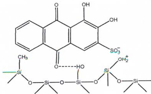
Gambar 7. Interaksi antara HMS dengan ARS pada suasana asam.
