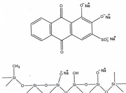
Gambar 8. Interaksi antara permukaan HMS dengan ARS pada suasana basa.
