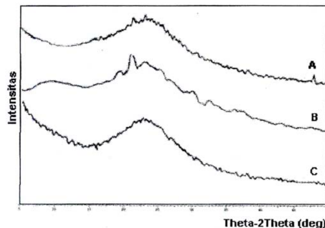
Gambar 4. Difraktogram sinar X, (A) HMS tanpa template , (B) HMS dengan template sebelum ekstraksi, (C) HMS setelah ekstraksi.
