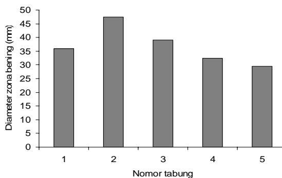
Gambar 2. Hasil pengujian aktivitas antibiotika dari mutan yang diperoleh.
