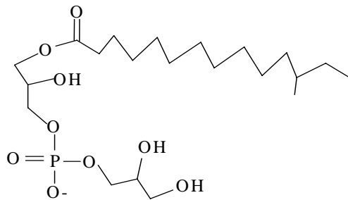
Gambar 3. Struktur kimia dari bacilycosin.
