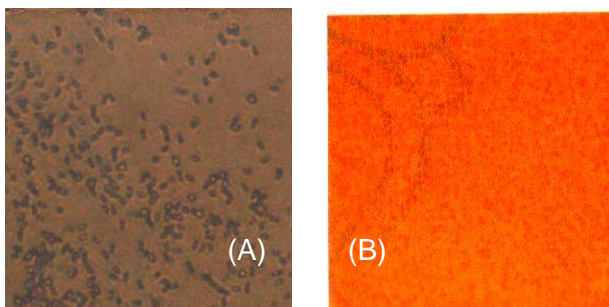
Gambar 6. Hasil pengamatan morfologi sel [(A). B. subtilis BAC4 dan (B). B. subtilis M10].
