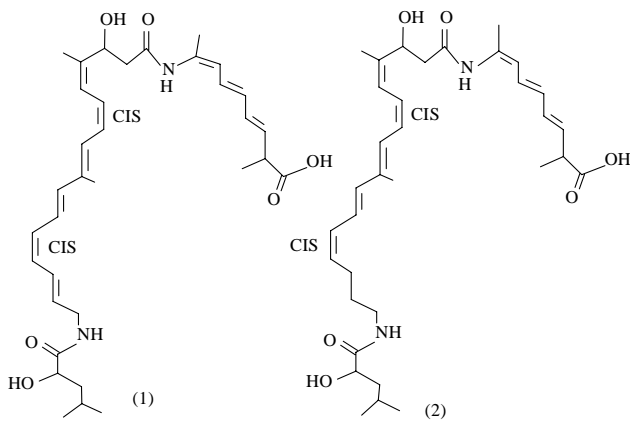
Gambar 4. Struktur kimia dari (1). basilaene dan (2). Dihydrobasilaene
