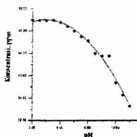
Gambar 1. Pengaruh pH terhadap konsentrasi emas
