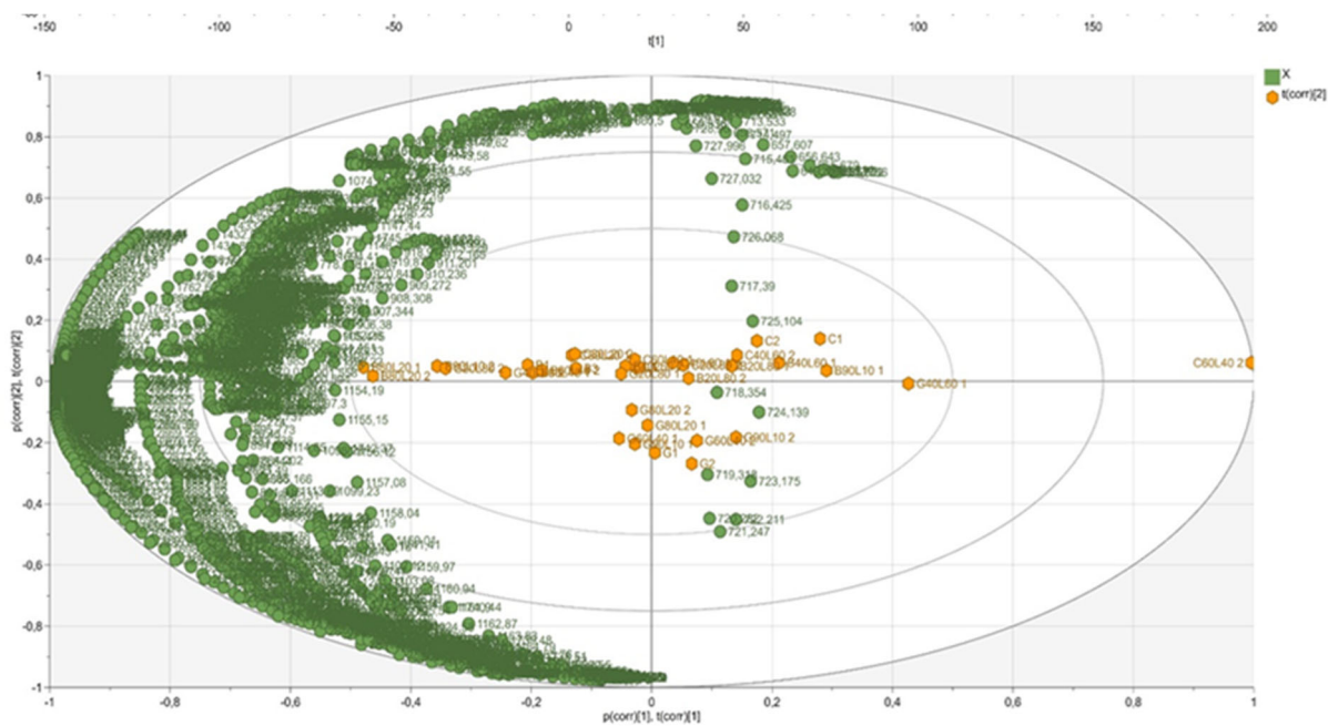
Fig S1. Bi plot FTIR
