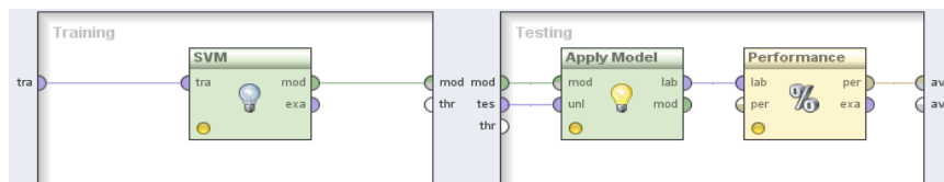
Gambar 7. Proses klasifikasi dengan support vector machine Rapid Miner 5.1
