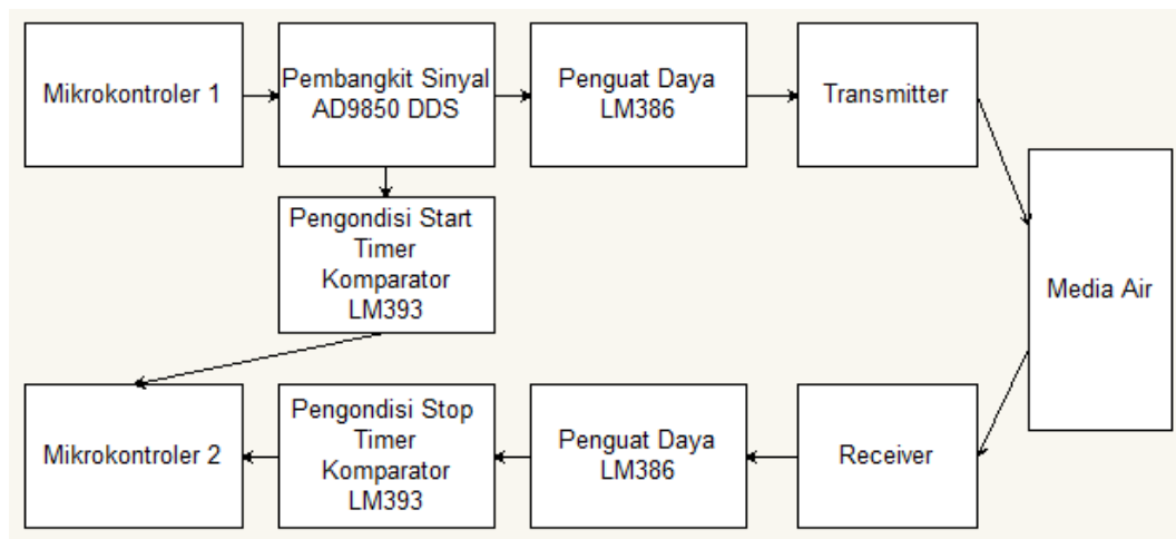
Gambar 1 Diagram blok sistem secara keseluruhan
