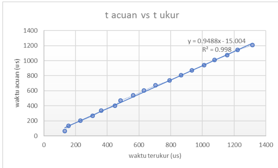
Gambar 14 Grafik perbandingan waktu acuan dengan waktu terukur
