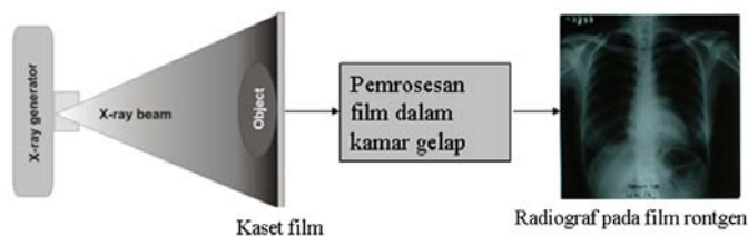
Gambar 1. Sistem Radiografi Konvensional
