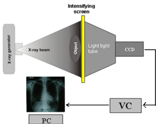
Gambar 2. Sistem RD menggunakan kamera CCD
