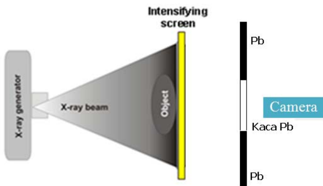
Gambar 5. Rancang bangun sistem RD berbasis kamera digital
