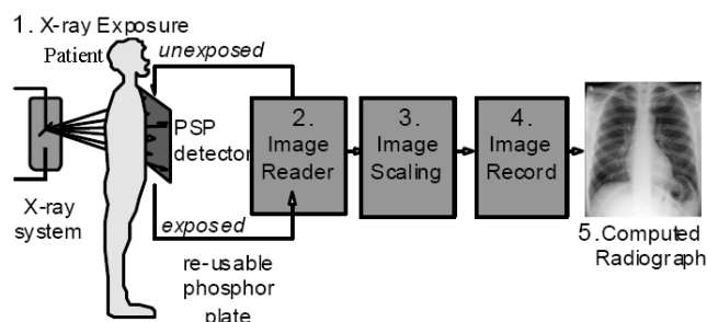
Gambar 3. Langkah siklus pencitraan sistem CR [5]
